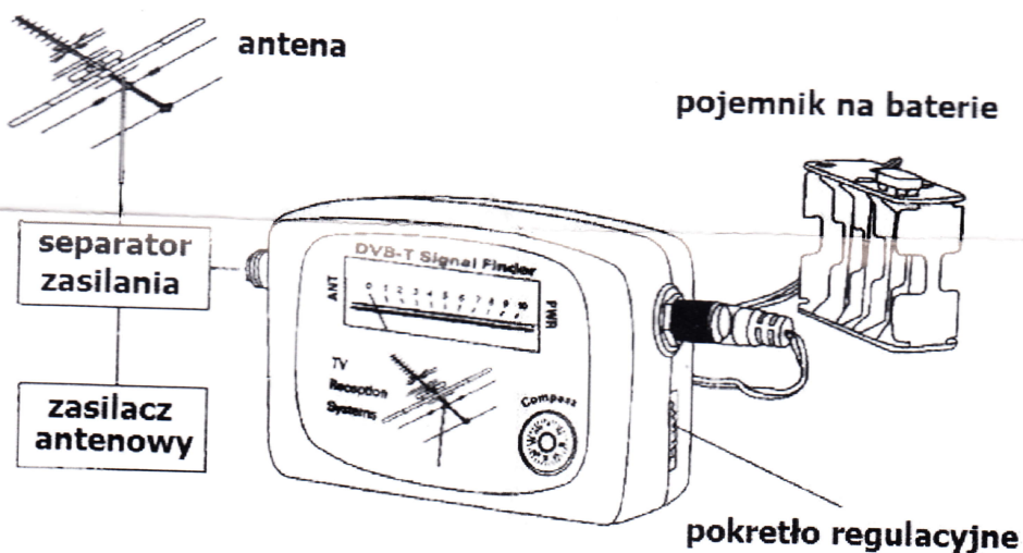
Rys. 2 Podłączenie miernika w przypadku anteny ze wzmacniaczem
