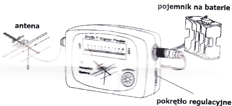
Rys. 1 Podłączenia miernika w przypadku anteny bez wzmacniacza
